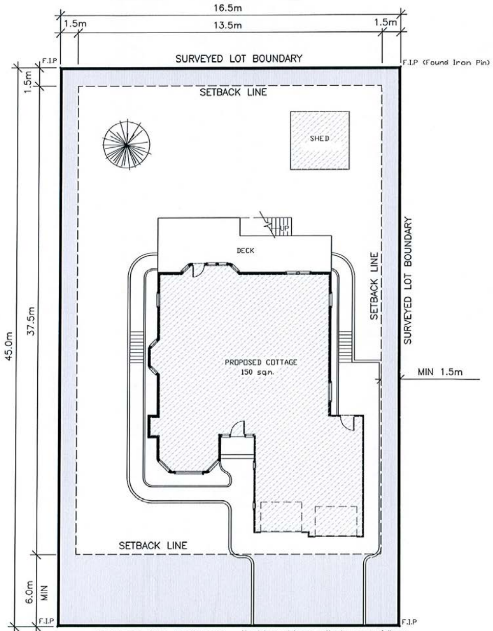
1 PLOT PLAN 5 N.T.S.
